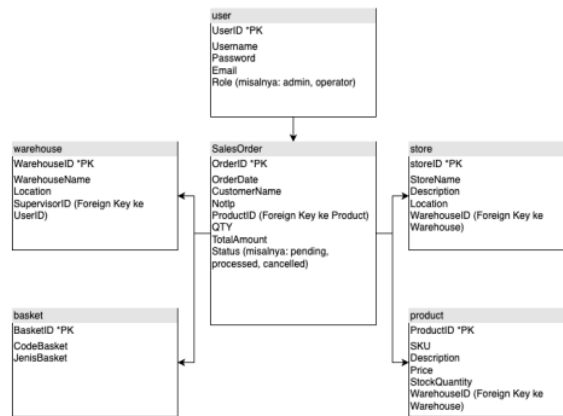
Gambar 8 Relasi Data
