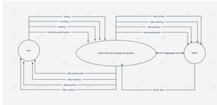
Gambar 4 DFD Lvl 0
