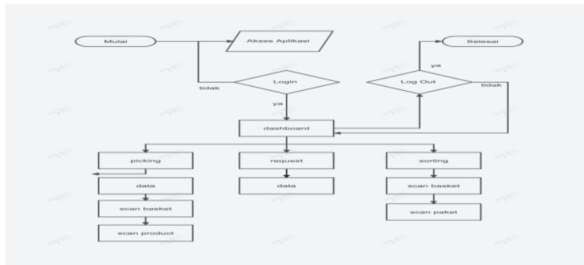
Gambar 3 Flowchart Sistem Aplikasi Mobile
