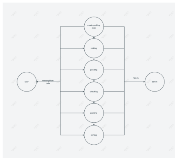
Gambar 5 DFD Lvl 1
