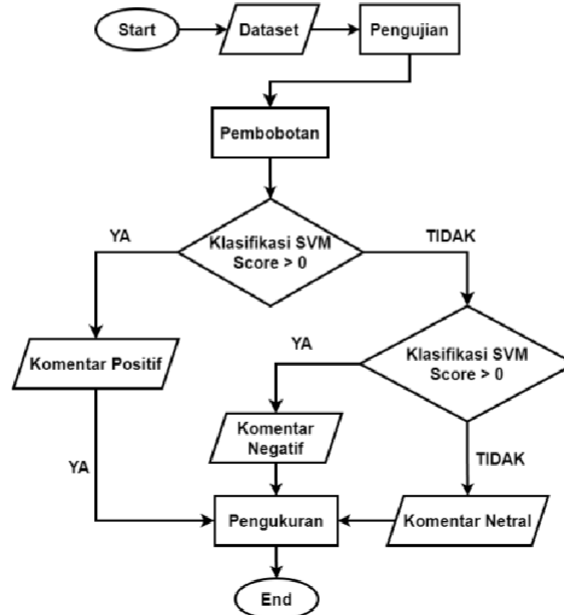
Gambar 1. Proses Klasifikasi SVM
