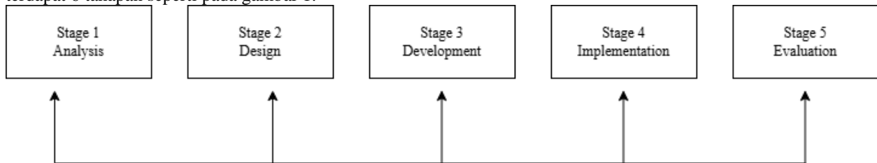
Gambar 1 Desain SDLC
