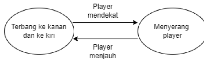
Gambar 5 FSM Enemy Fly A
