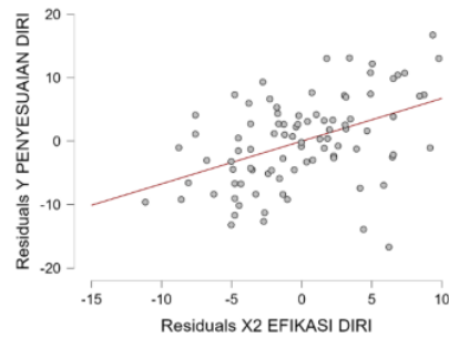
Gambar 3. Grafik Uji Linieritas (2)
