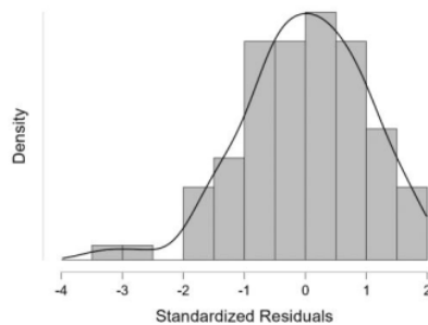
Gambar 1. Grafik Uji Normalitas
