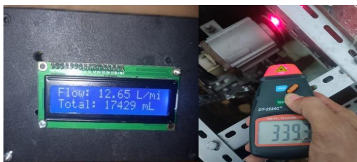
Gambar 15. Debit air dan RPM Generator
