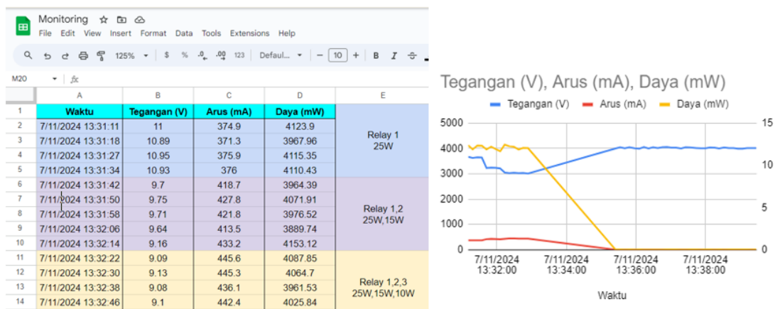
Gambar 21. Hasil Monitoring pada Google Sheets
