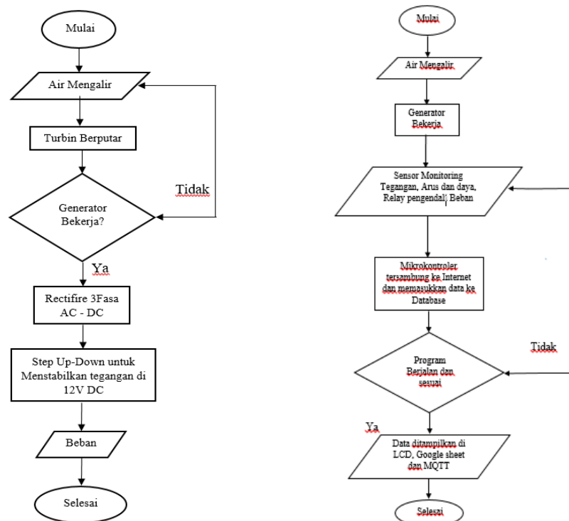
Gambar 11. Flowchart cara kerja sistem konversi energy listrik dan Sistem Monitoring dan kendali Beban PLTMH
