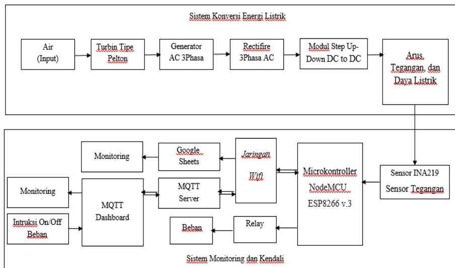
Gambar 7. Diagram Blok sistem konversi energi dan sistem monitoring dan pengendalian beban
