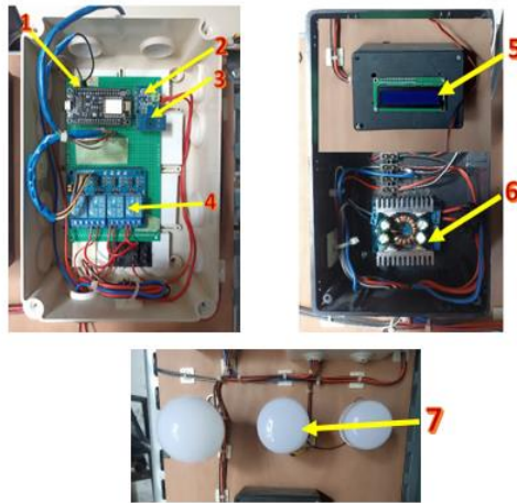
Gambar 14. Perakitan Komponen
