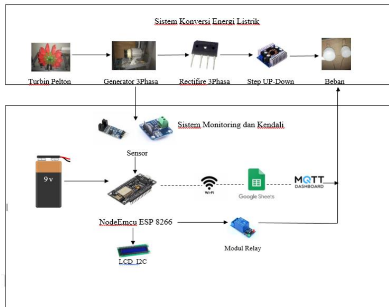
Gambar 10. Skema pembangkit listrik tenaga mikrohidro berbasis IoT
