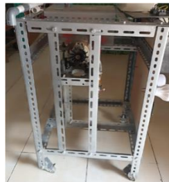
Gambar 12. Pondasi PLTMH
