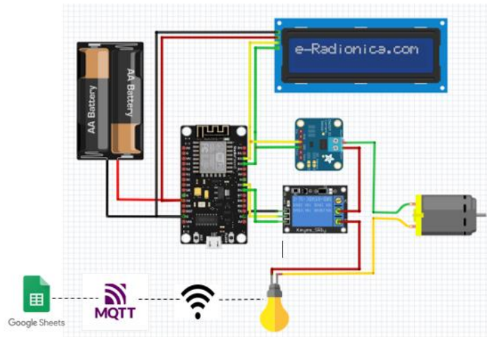
Gambar 8. Rangkaian sistem monitoring kendali beban
