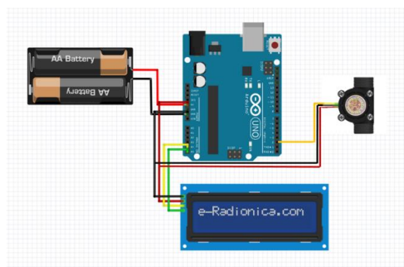
Gambar 9. Rangkaian untuk pembacaan flow air
