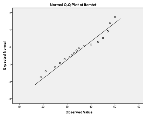
Gambar 1. Uji Normalitas
