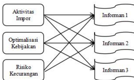
Gambar 2. Komponen Pertanyaan
