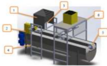
Gambar 2 Mesin Tabur Wijen Konsep A
