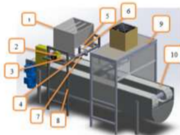
Gambar 3 Mesin Tabur Wijen Konsep B
