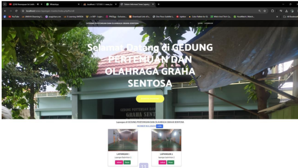
Gambar 3.1 Halaman Utama
