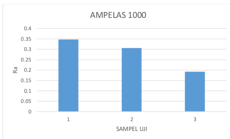
Gambar 13. Diagram uji kekasaran sampel menggunakan ampelas 1000
