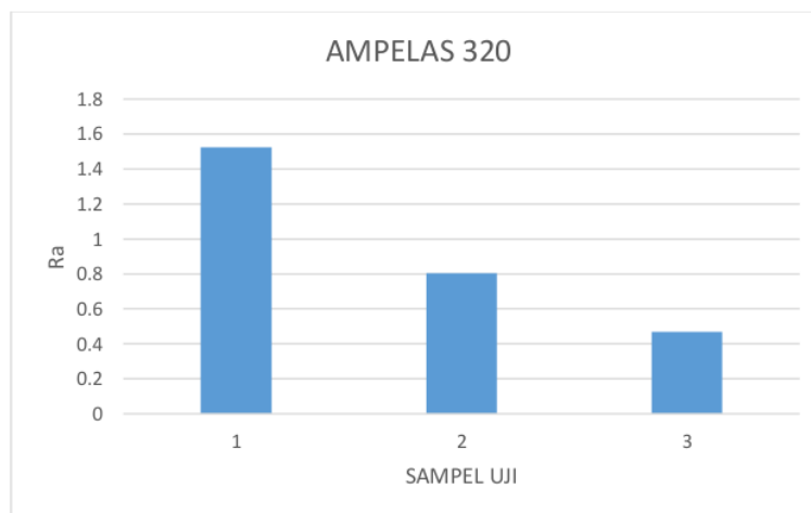
Gambar 12. Diagram uji kekasaran sampel menggunakan ampelas 320
