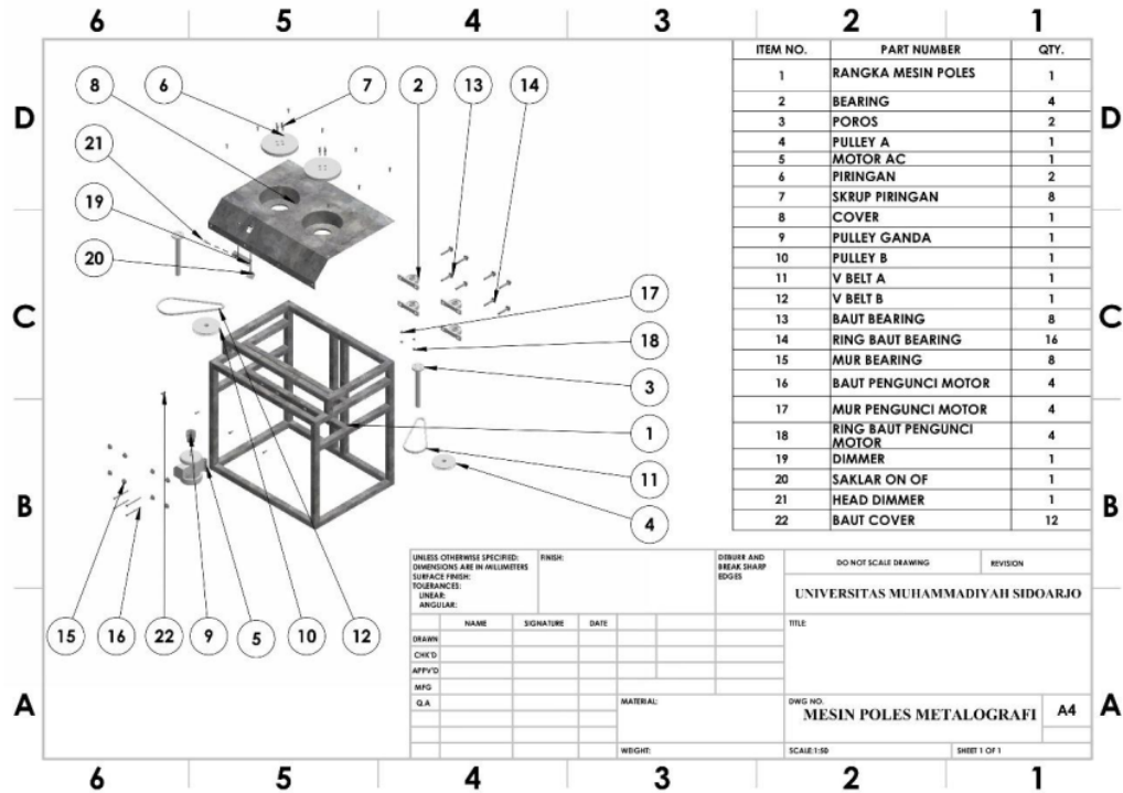
Gambar 6. Detail Desain Mesin Poles
