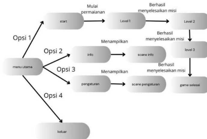
Gambar 3. Diagram Finite State Pada Menu Utama
