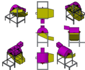
Gambar 4. Komponen Mesin
