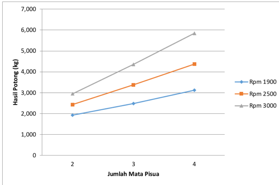
Gambar 12. Grafik Hasil Potong Mesin Pencacah Rumpun
