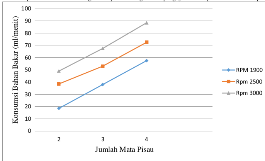
Gambar 13. Grafik Bahan Bakar Mesin Pencacah Rumput
