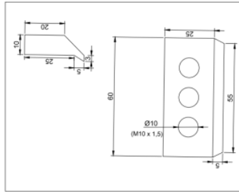
Gambar 3. Mata Pisau
