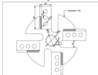
Gambar 2. Desain Support Pisau Pencacah
