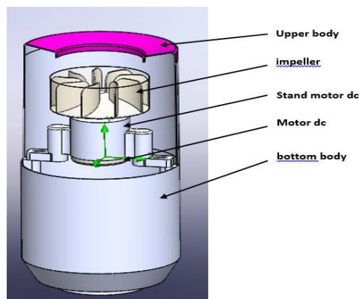
Gambar 3. Hasil Konsep Desain Blade Pengering Tangan
