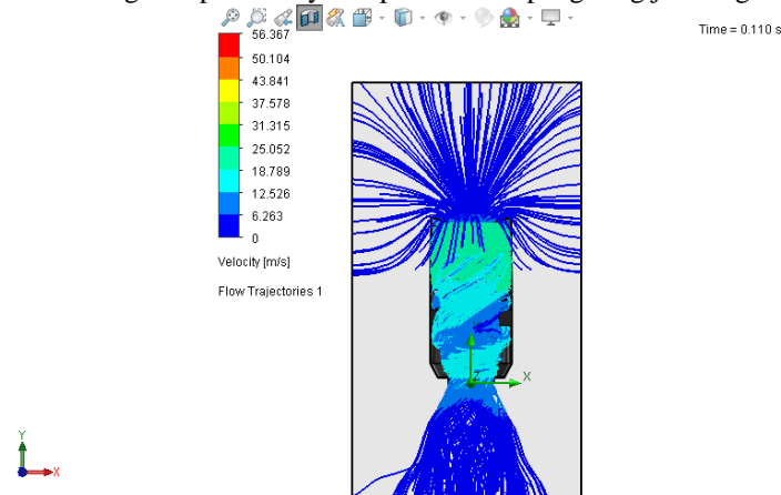
Gambar 5. Simulasi Velocity
