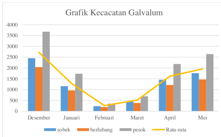
Gambar 2. Grafik Kecacatan Galvalum
