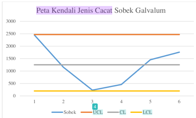
Gambar 4. Peta Kendali Jenis Cacat Sobek Galvalum
