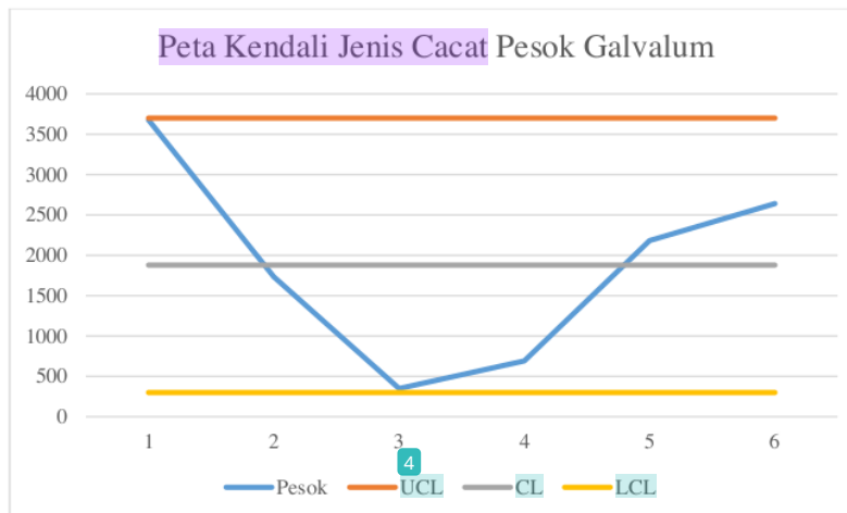
Gambar 5. Peta Kendali Jenis Cacat Pesok Galvalum
