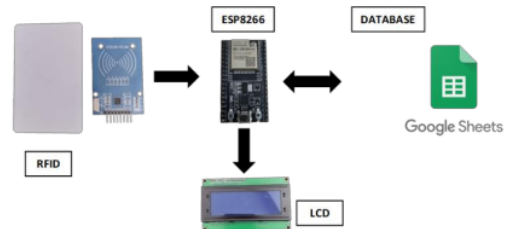
Gambar 3. Desain Rancang Alat
