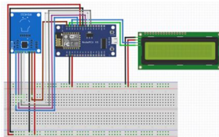
Gambar 4. Rangkaian Skematik Keseluruhan
