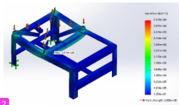
Gambar 8. Simulasi Tegangan ( von mises stress )
