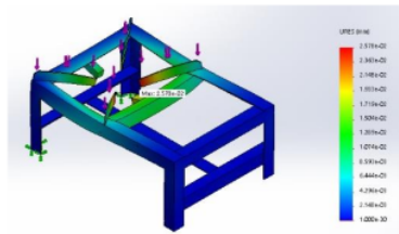
Gambar 9. Simulasi Lendutan ( displacement )
