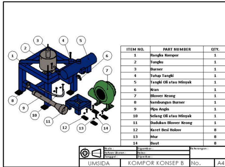
Gambar 7. Komponen Kompor Burner Konsep B
