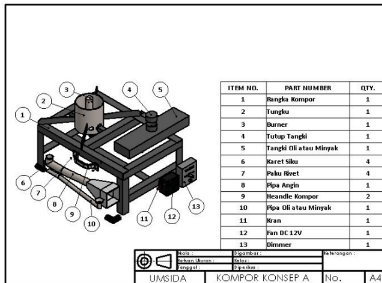
Gambar 6. Komponen Kompor Burner Konsep A
