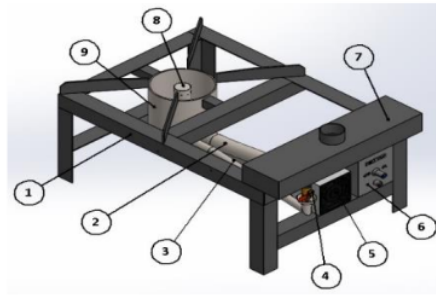
Gambar 4. Konsep A Kompor Burner
