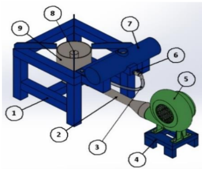
Gambar 5. Konsep B Kompor Burner
