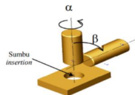
Gambar 3. Prinsip Rotasi Simetri Alpa dan Beta
