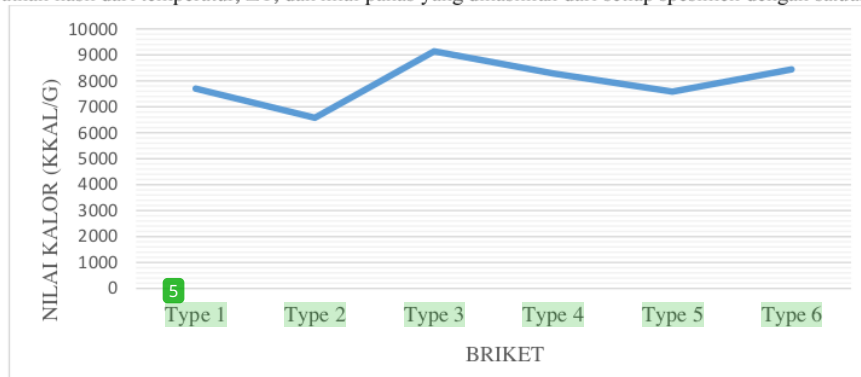
Gambar 6 Grafik Uji Nilai Kalor Arang Briket Sekam Padi dan Batang Jerami Padi
