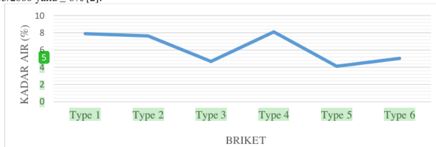
4 Gambar 5 Grafik Uji Kadar Air Arang Briket Sekam Padi dan Batang Jerami Padi
