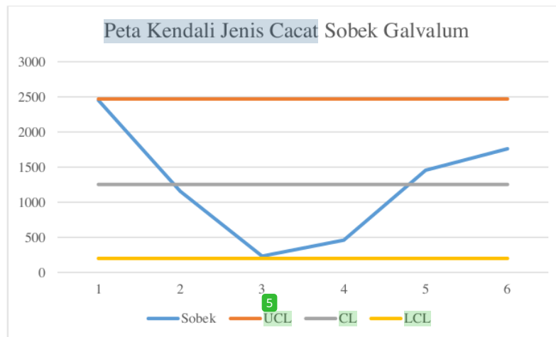
Gambar 4. Peta Kendali Jenis Cacat Sobek Galvalum
