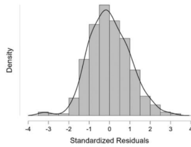
Gambar 1. Uji normalitas
