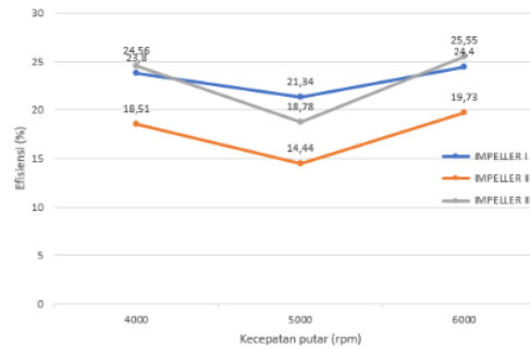
Gambar 7. Grafik Efisiensi dan Kecepatan Putar (Rpm)
