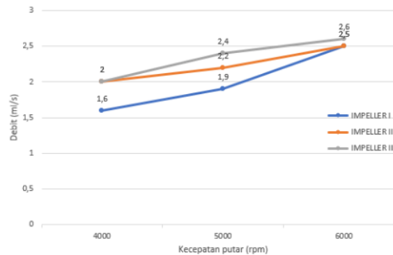
Gambar 6. Grafik Debit dan Kecepatan Putar (Rpm)
