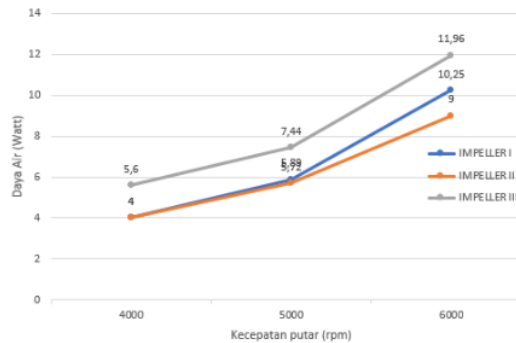
Gambar 7. Grafik Daya Air dengan Kecepatan Putar (Rpm)
