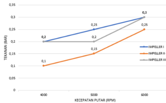
Gambar 5. Grafik Rpm dan Tekanan (Bar)
