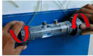
Gambar 4. pemasangan spesimen
