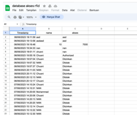
Gambar 6. Pengujian Pengiriman Data ke Google Spreadsheet
