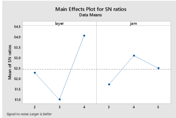
Gambar 12. Grafik SN ratio Pengujian tekuk
