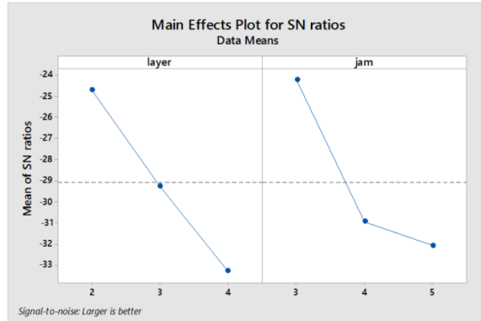
Gambar 11. Grafik SN ratio Pengujian tarik
