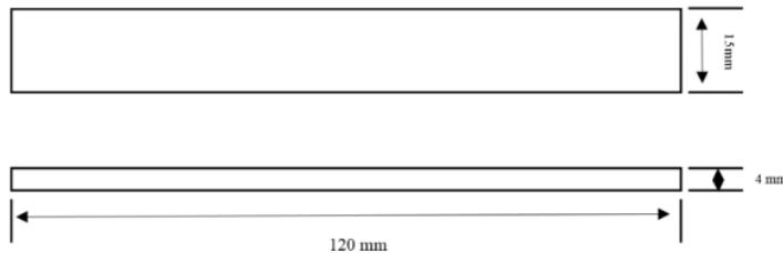
Gambar 4. Spesimen Uji tekuk ASTM D790
