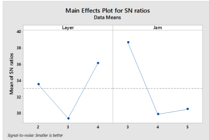
Gambar 13. Grafik SN ratio Pengujian kerataan permukaan
