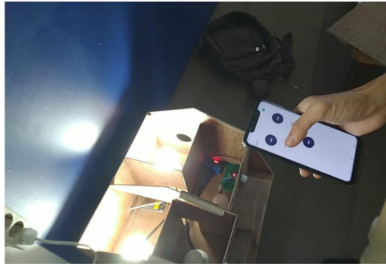
Gambar 8. Tampilan Demo Aplikasi Blynk
