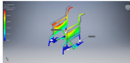
Gambar 13 Hasil analisa perpindahan ( displacement ) pada body konsep A
