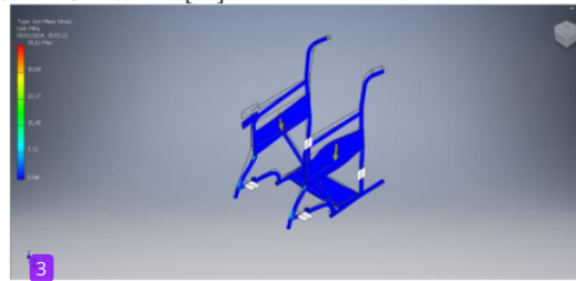
Gambar 14 Tegangan von mises pada body konsep B
