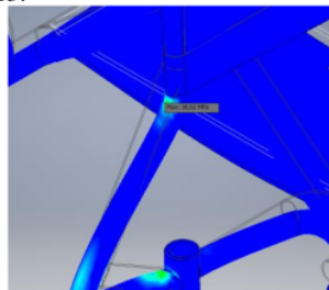
Gambar 15 Tegangan maksimal von mises pada body konsep B
