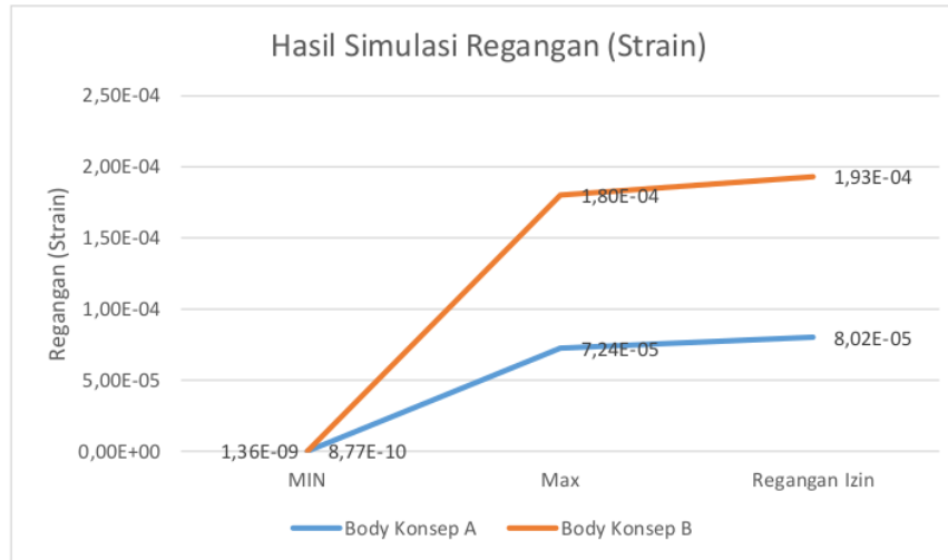
Gambar 22 Grafik hasil simulasi regangan ( strain )
