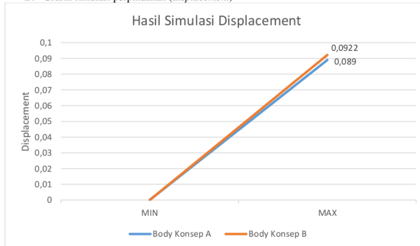
Gambar 21 Grafik hasil simulasi displacement
