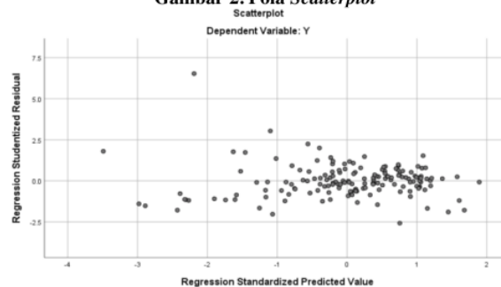
Gambar 2. Pola Scatterplot
