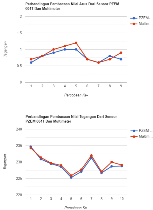
Gambar 6. Grafik Perbandingan Pembacaan Arus Sensor PZEM-004T dengan Multimeter
