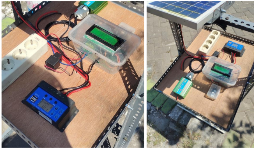
Gambar 4. Proses Pengisian Pada Panel Surya
