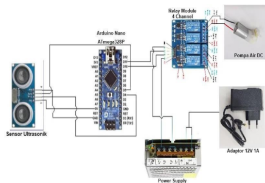
Gambar 3. Rangkaian Peralatan Pencuci Tangan
