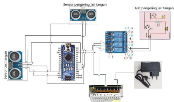
Gambar 5. Rangkaian Peralatan Pengering tangan
