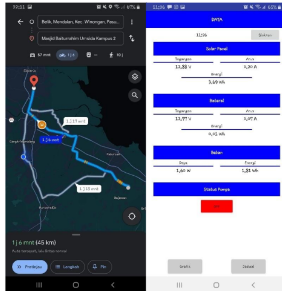
Gambar 10. Pengujian Lokasi Ketiga
