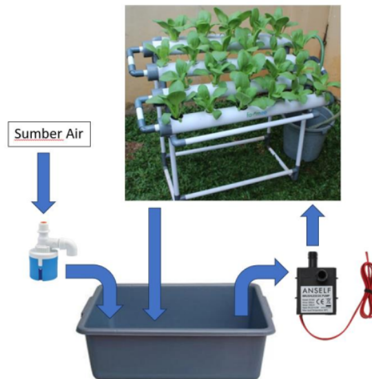
Gambar 3. Visualisasi Desain Alat
