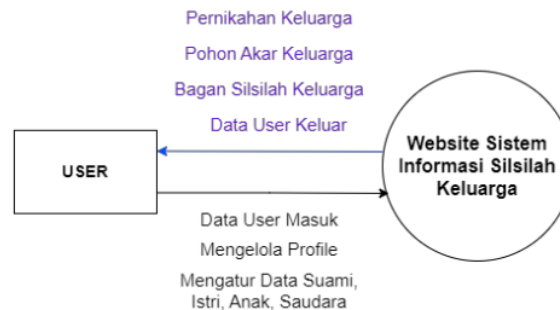
Gambar 3. Diagram Konteks DFD
