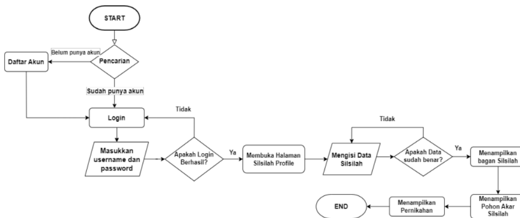
Gambar 2. Flowchart Silsilah Keluarga
