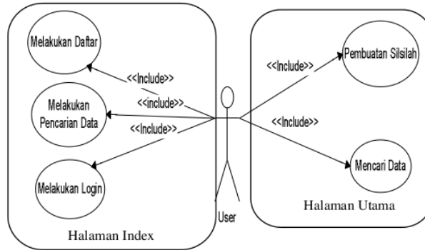
Gambar 5. Use Case Diagram Silsilah Keluarga
