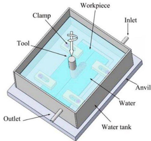
Gambar 3. Layout pengelasan UWFSW
