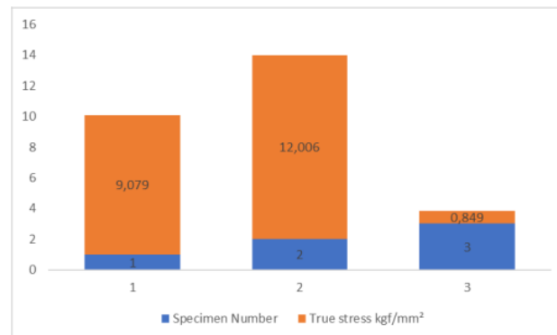
Gambar 5. Hasil uji Tarik masing-masing spesimen UFSW
