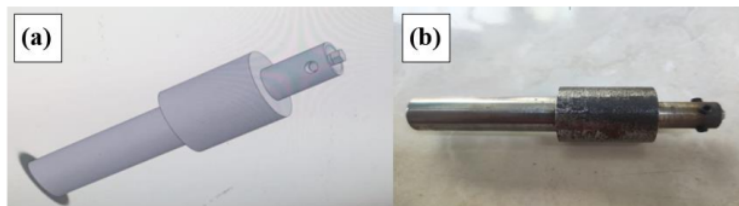
Gambar 1. Tool UWFSW: (a) desain tool dan (b) manufaktur tool
