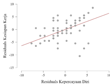
Gambar 1 Grafik Scatter Plot Sebaran Data
