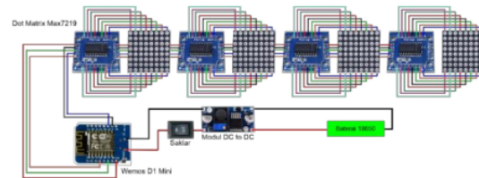
Gambar 4. Perancangan Alat
