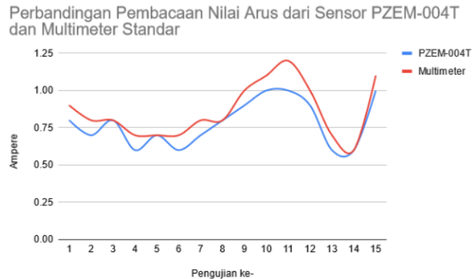
Gambar 6. Grafik Perbandingan Pembacaan Arus Sensor PZEM-004T dengan Multimeter
