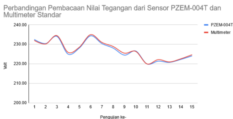
Gambar 5. Grafik Perbandingan Pembacaan Tegangan Sensor PZEM-004T dengan Multimeter
