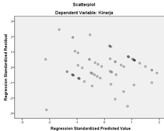
Gambar 3. Uji Heteroskedastisitas
