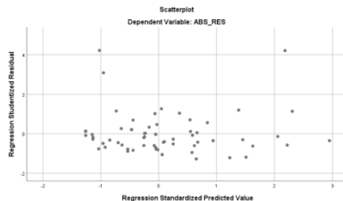
Gambar 3. Uji Heteroskedastisitas
