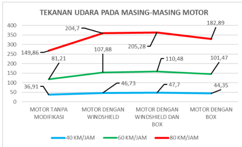
GRAFIK 1.2 FORCE (TEKANAN UDARA) MASING-MASING MOTOR
