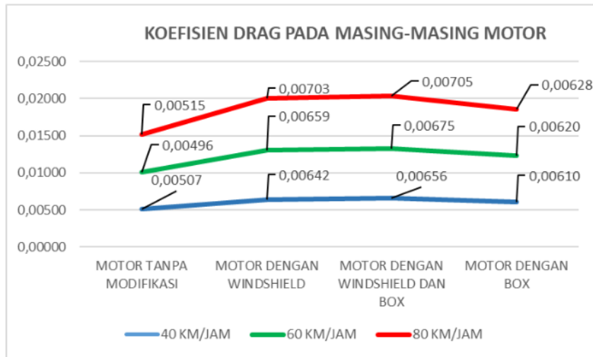
GRAFIK 1.1 KOEFISIEN DRAG MASING-MASING MOTOR
