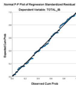
Gambar 1. Uji Normalitas
