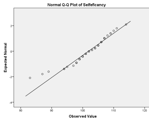
Gambar 1. Grafik Normalitas
