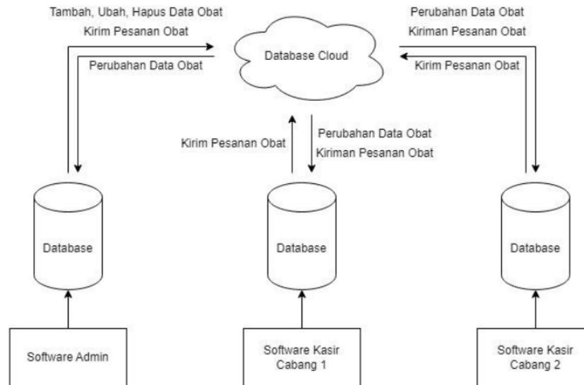
Gambar 8. Implementasi Database
