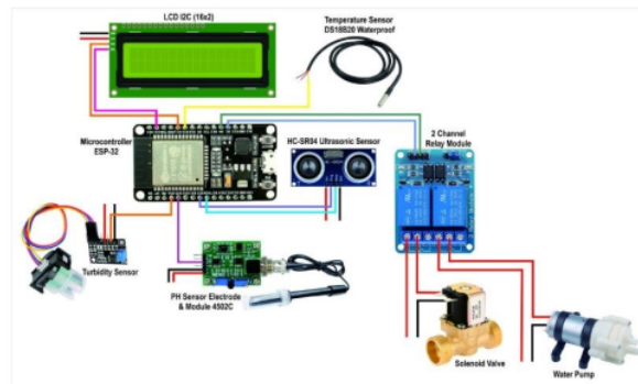
Gambar 3. Diagram Pengkabelan
