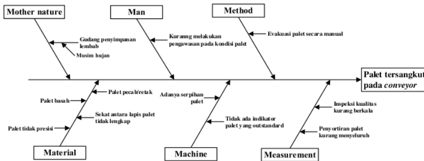
Gambar 1. Diagram tulang ikan palet tersangkut di conveyor
