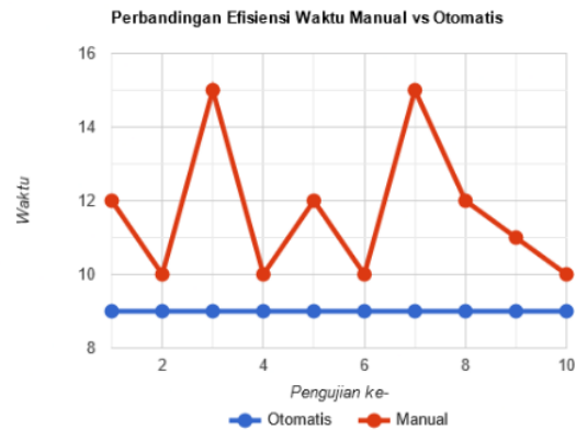
Gambar 6. Grafik Perbandingan Waktu Pengecatan Otomatis dan Manual
