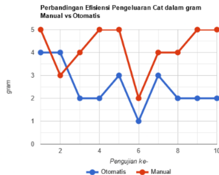
Gambar 7. Grafik Perbandingan Keluaran Cat dari Proses Pengecatan Otomatis dan Manual
