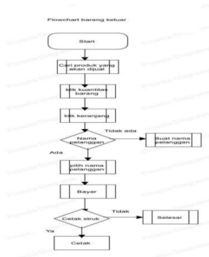
Gambar 2 Flowchart barang keluar
