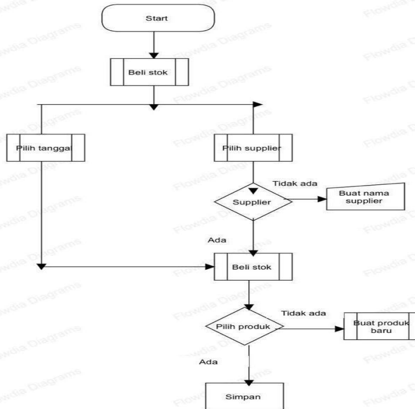
Flowchart pencatatan barang datang
