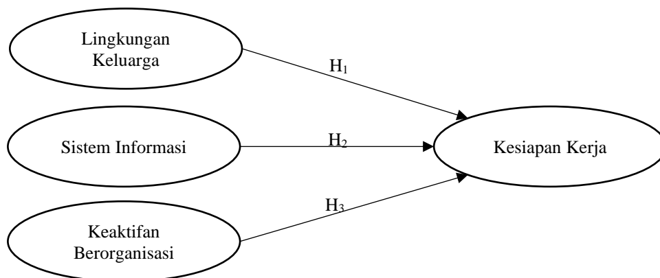
Gambar 4 Kerangka Konseptual
