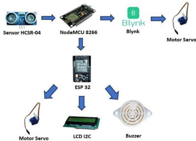
Gambar 1. Blok Diagram Sistem
