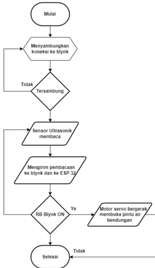
Gambar 3. Diagram alir pertama sistem kontrol program
