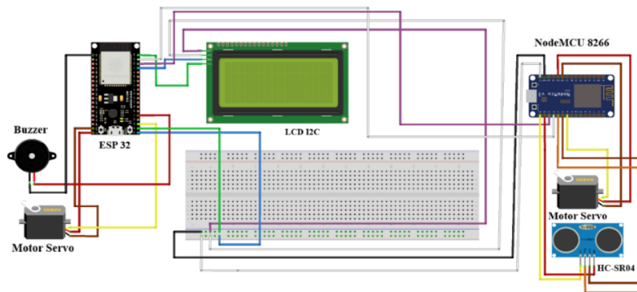
Gambar 2. Desain Pengkabelan
