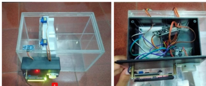
Gambar 5. Realisasi Alat
