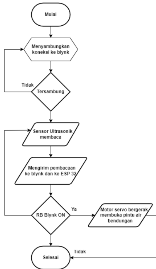
Gambar 4. Diagram alir kedua sistem pemantauan program
