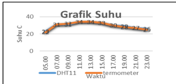
Gambar 6. Grafik Suhu Antara Sensor DHT11 dengan Thermometer Digital
