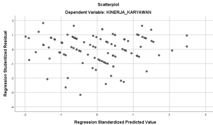
Gambar 3.2 Uji Heteroskedastisitas Sumber: Proses Data (2023)
