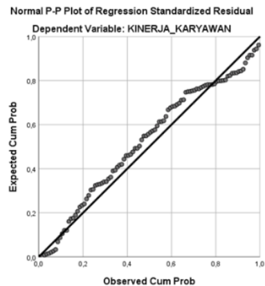
Gambar 3.1 Uji Normalitas Scatterplot Sumber: Proses data (2023)
