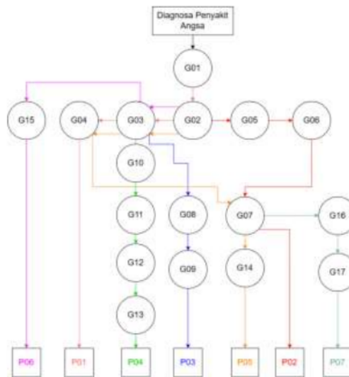
Gambar 3. Pohon Keputusan
